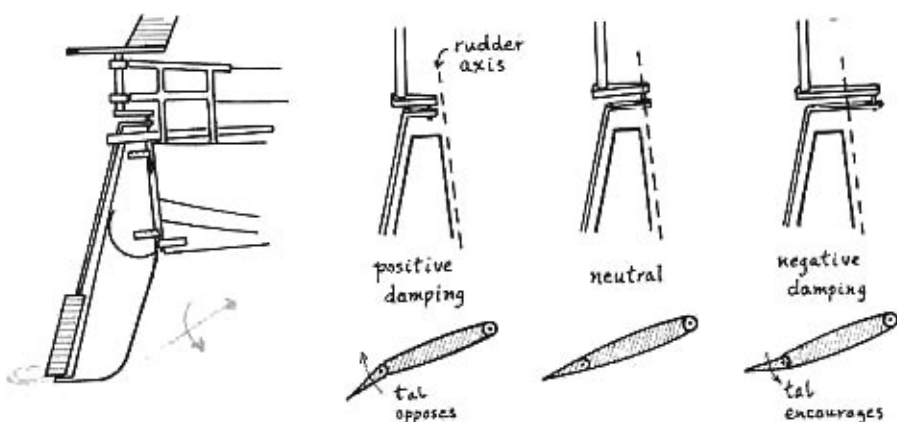
7-9. Feedback linkages for servo tab.
